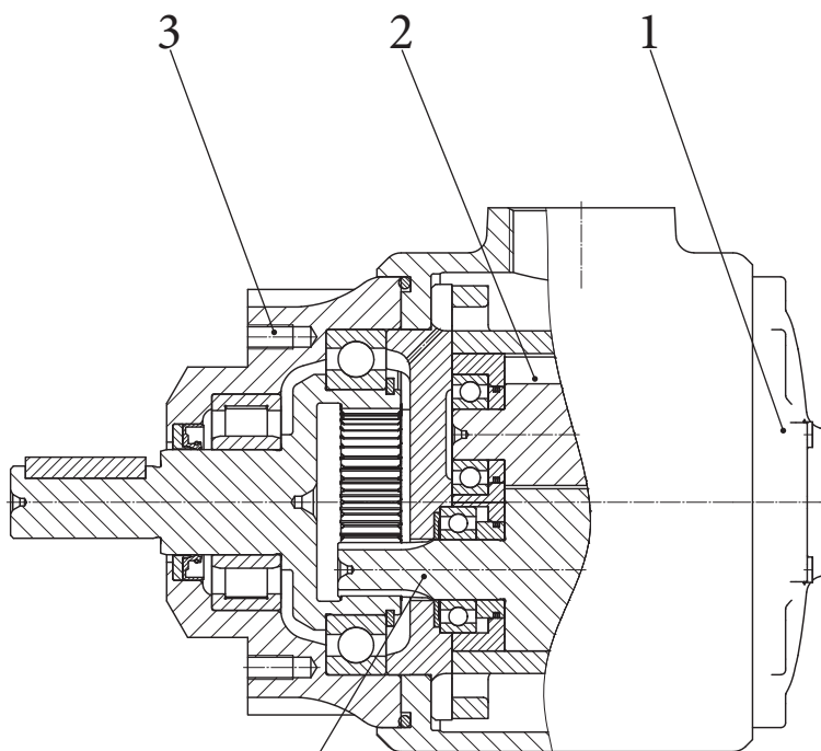
Antriebsrotor unten
